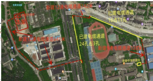
管道示意图
