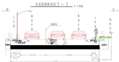
管道断面图
